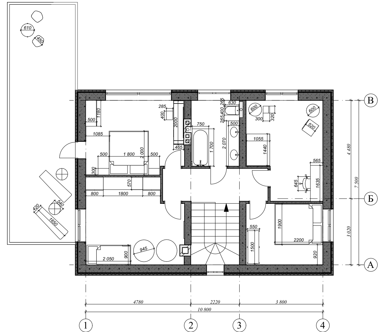
2 поверх
