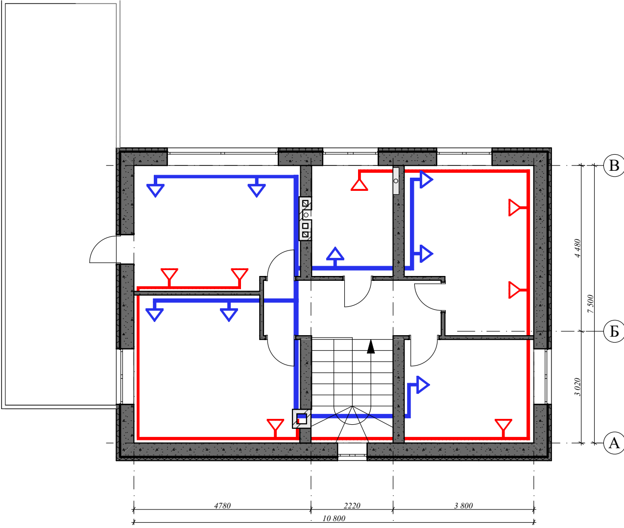
2 поверх
