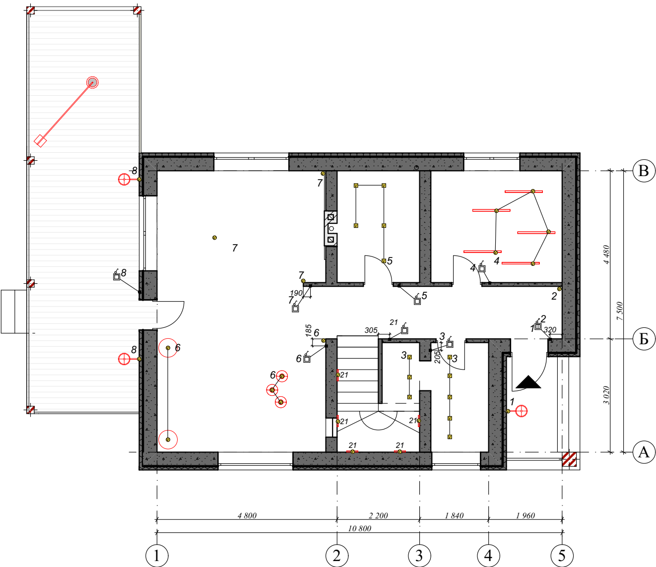
1 поверх
