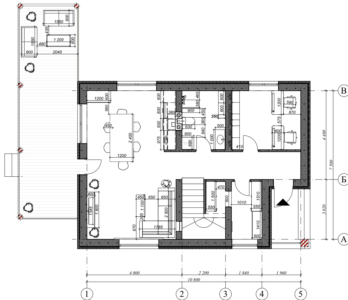
1 поверх
