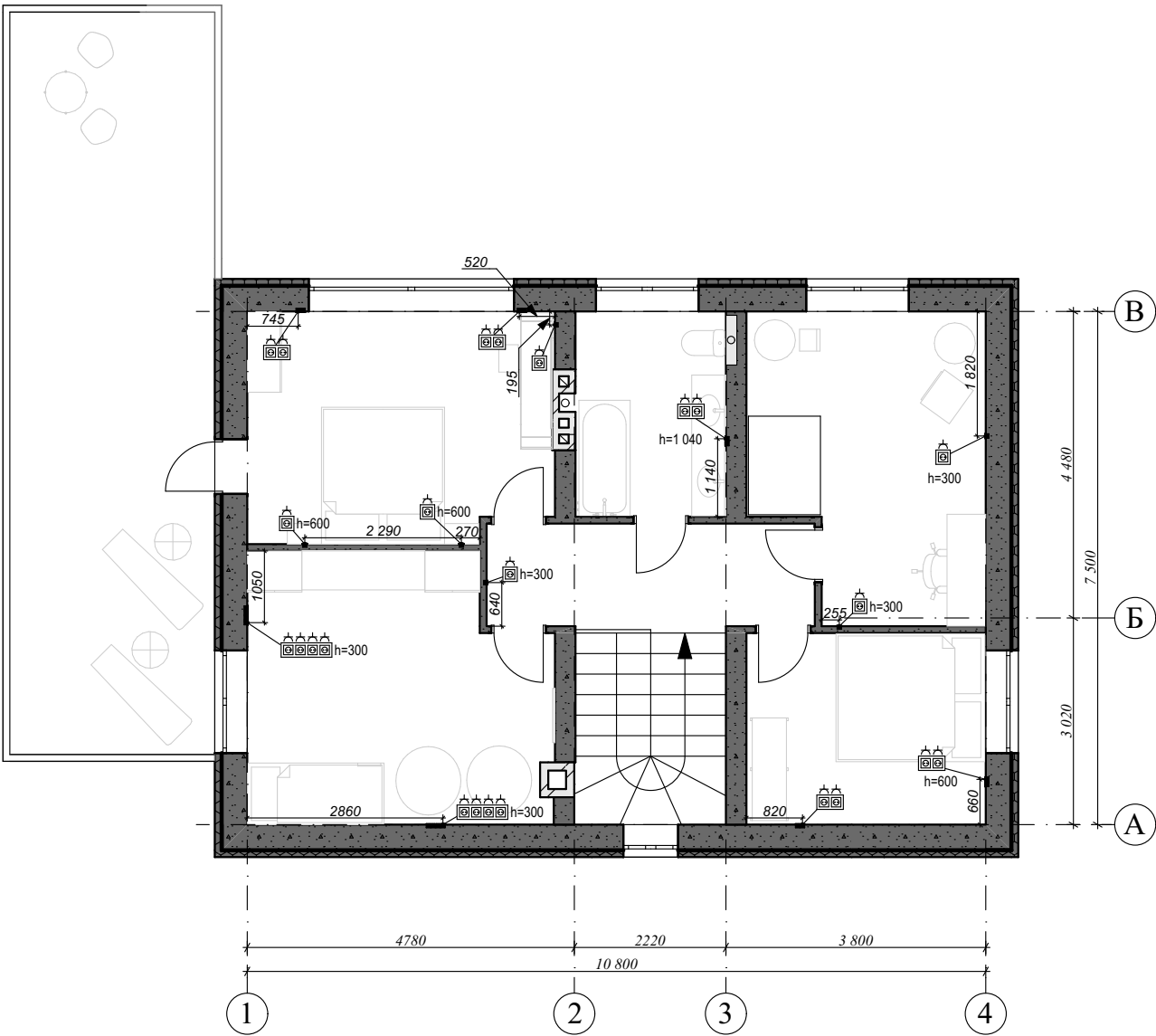
2 поверх
