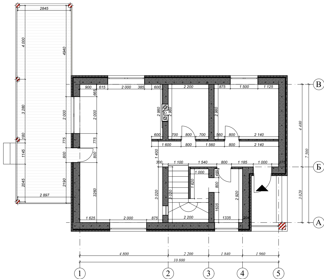
1 поверх
