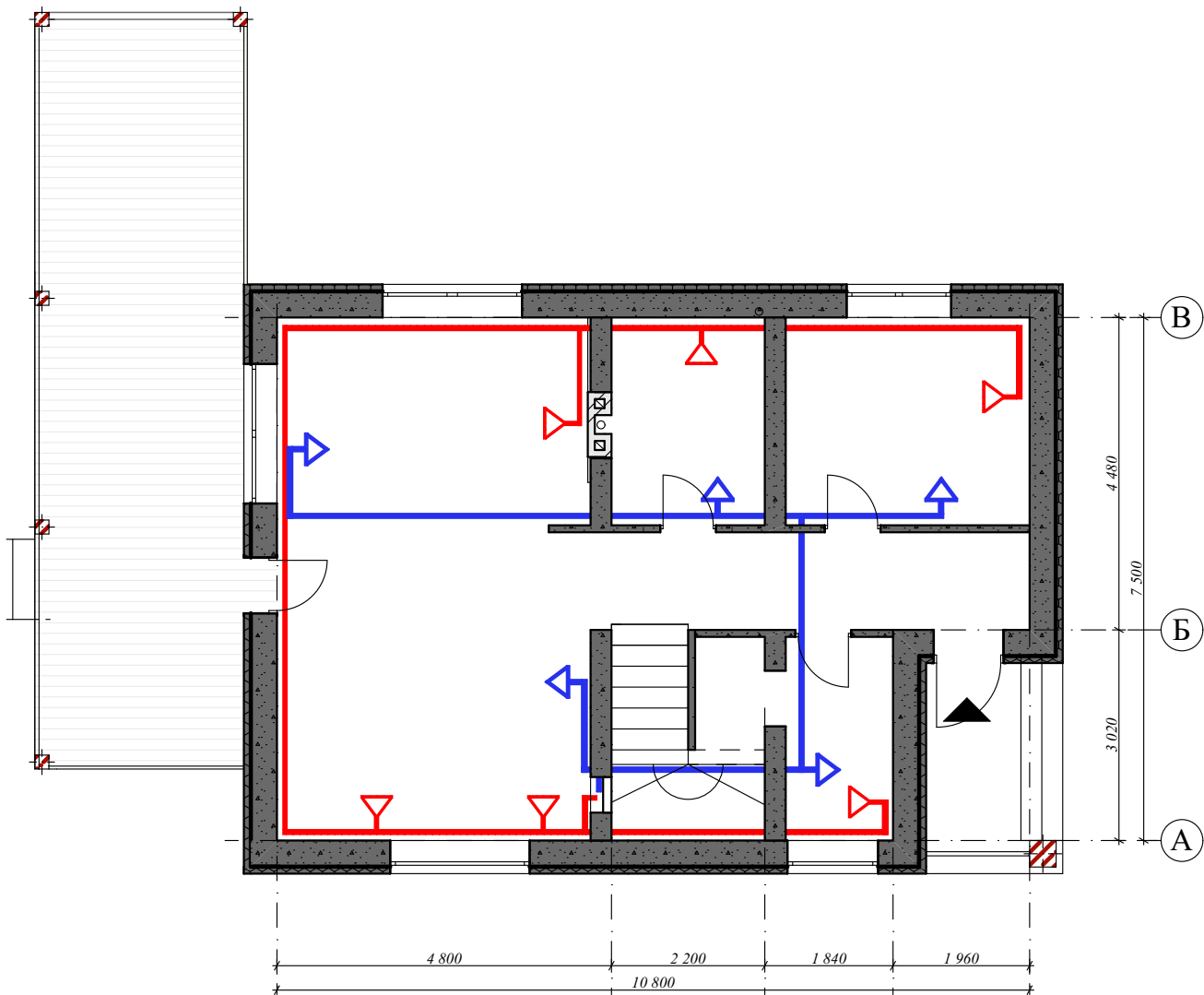
1 поверх
